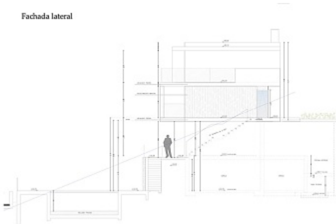
Fachada lateral
